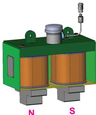
W1B12X24 Bi Polar Unit
